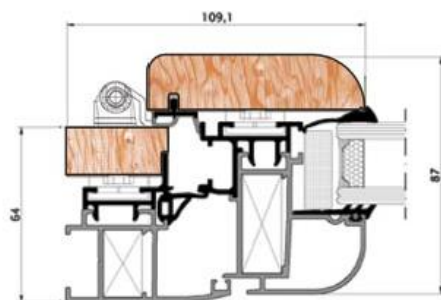
nodo laterale
